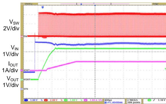
Time 400μs/div
