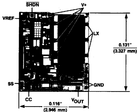
MAX738/MAX758
